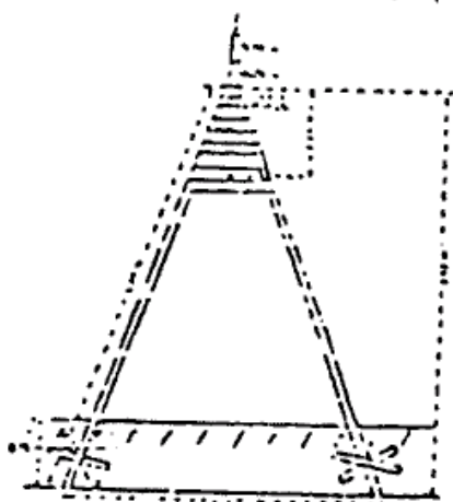
二三等點尋常方錐形木標
